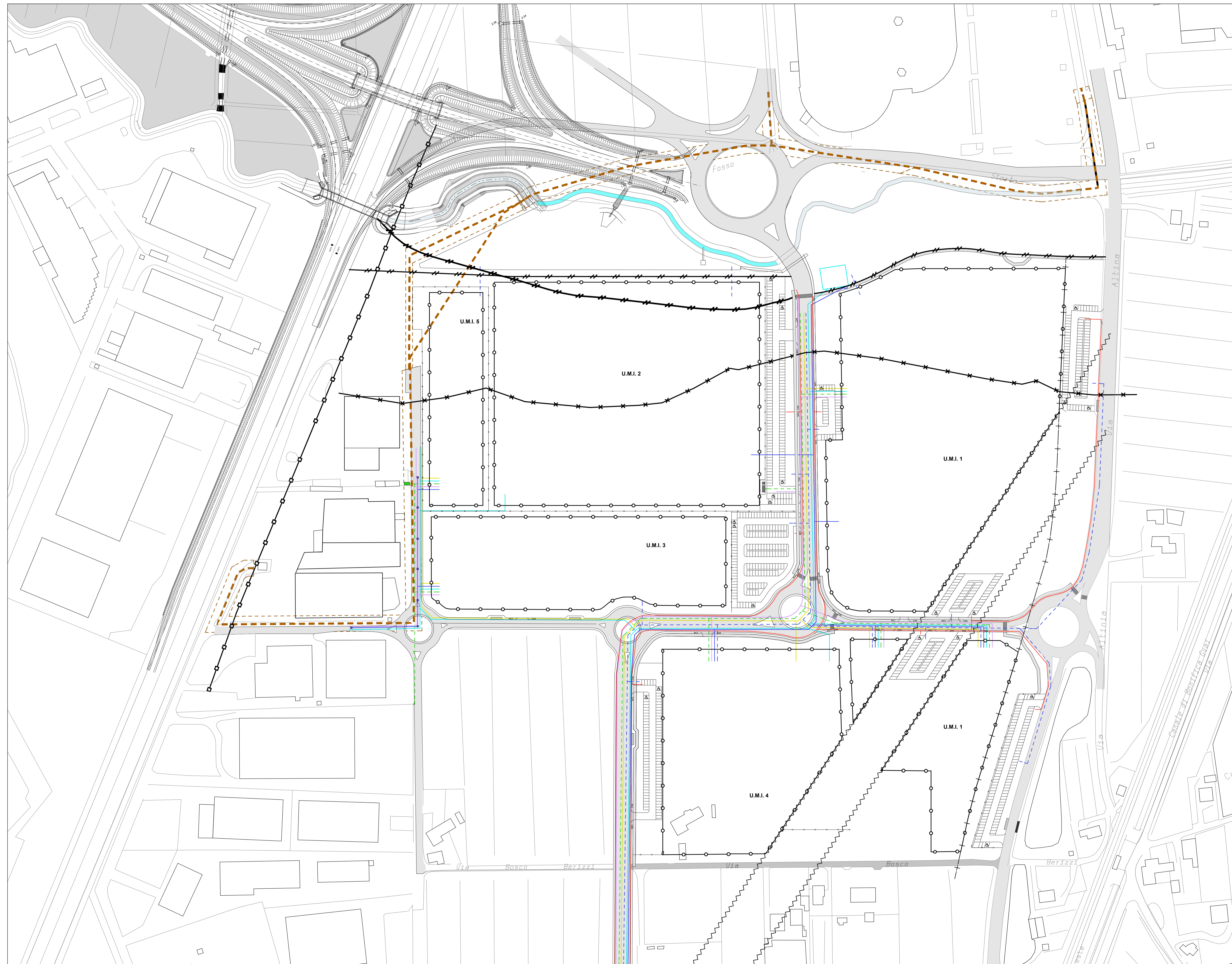
TRACCIATI RETI SOTTOSERVIZI - STATO DI PROGETTO
