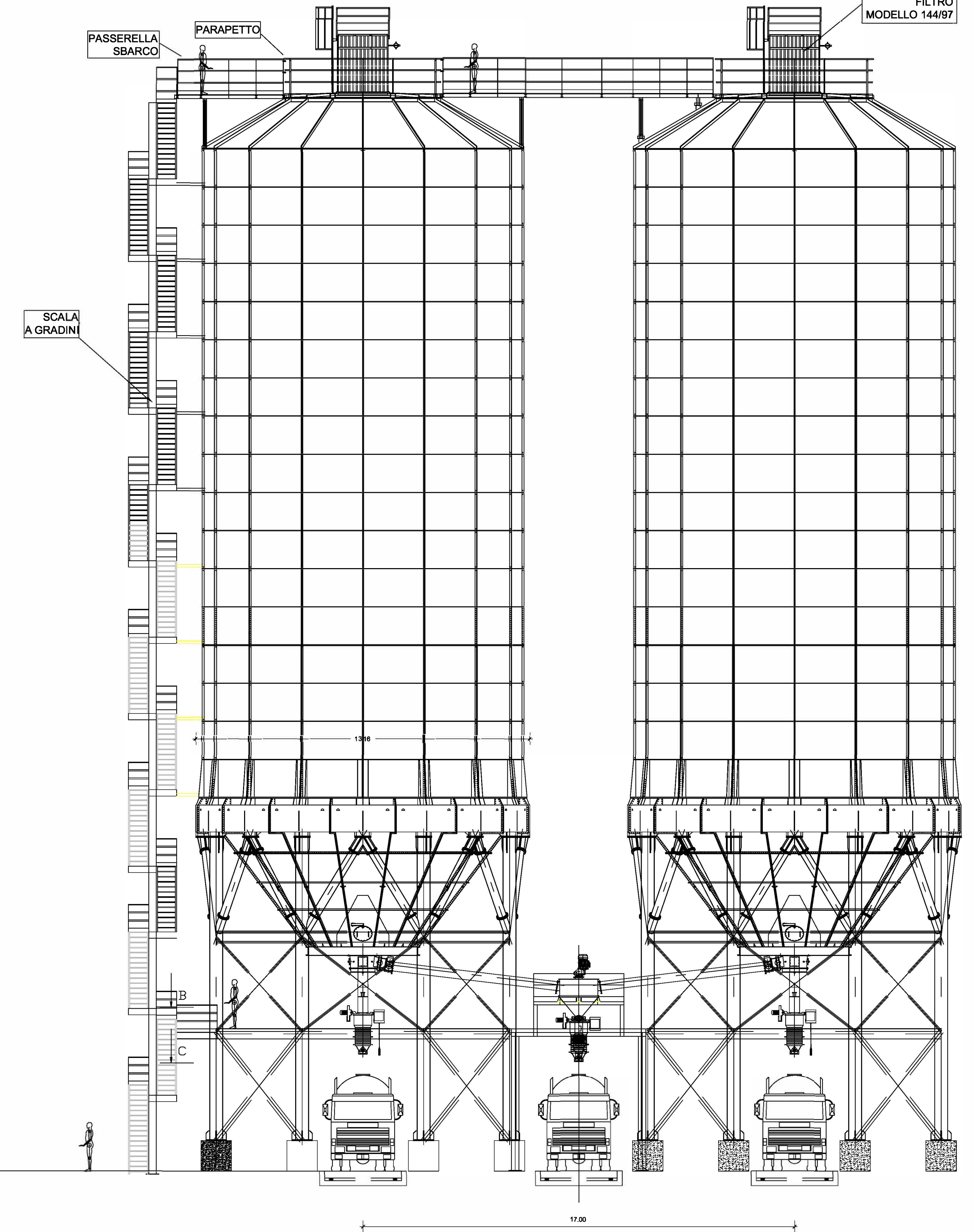
VISTA FRONTALE SCALA 1:125
