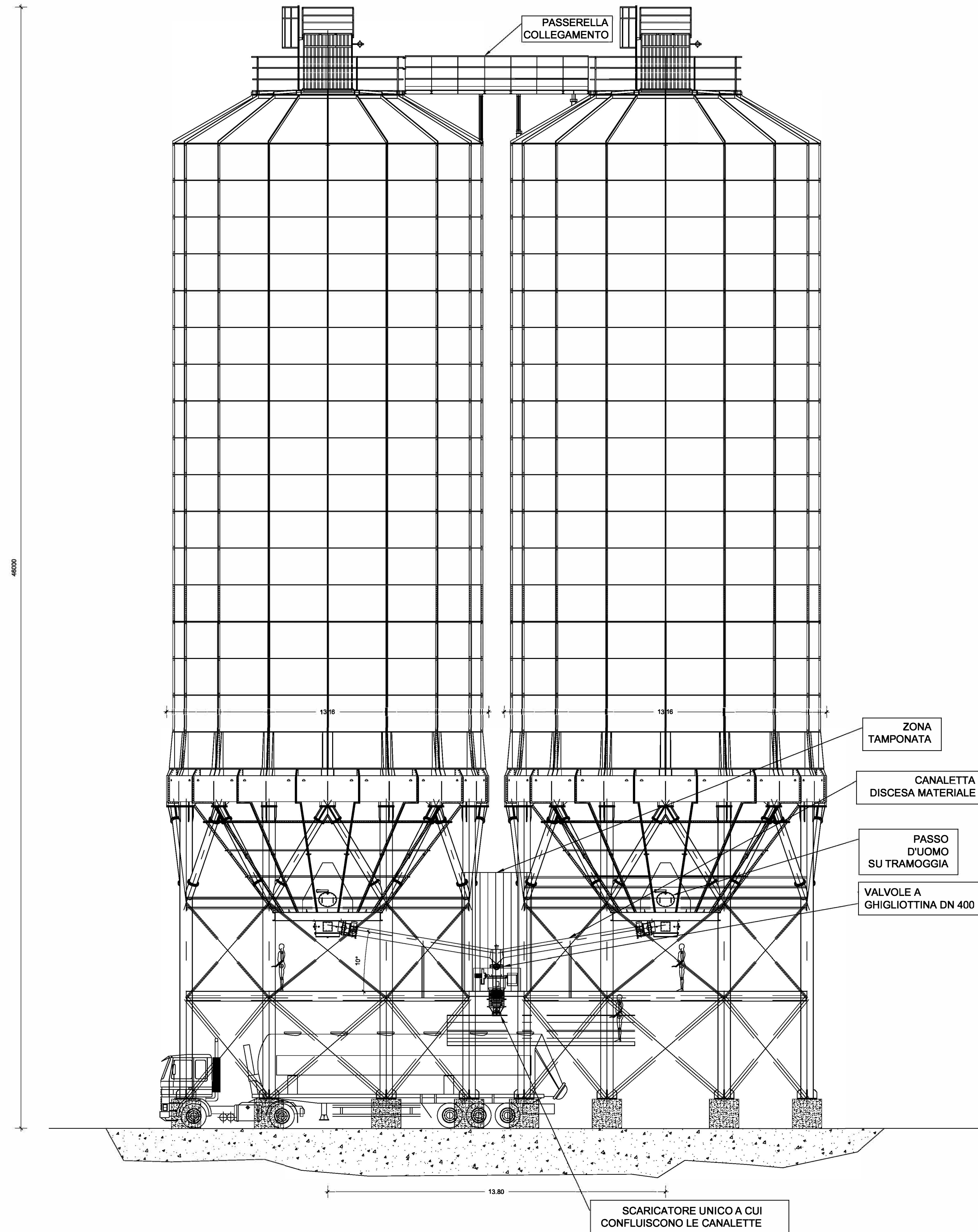
VISTA LATERALE SCALA 1:125
