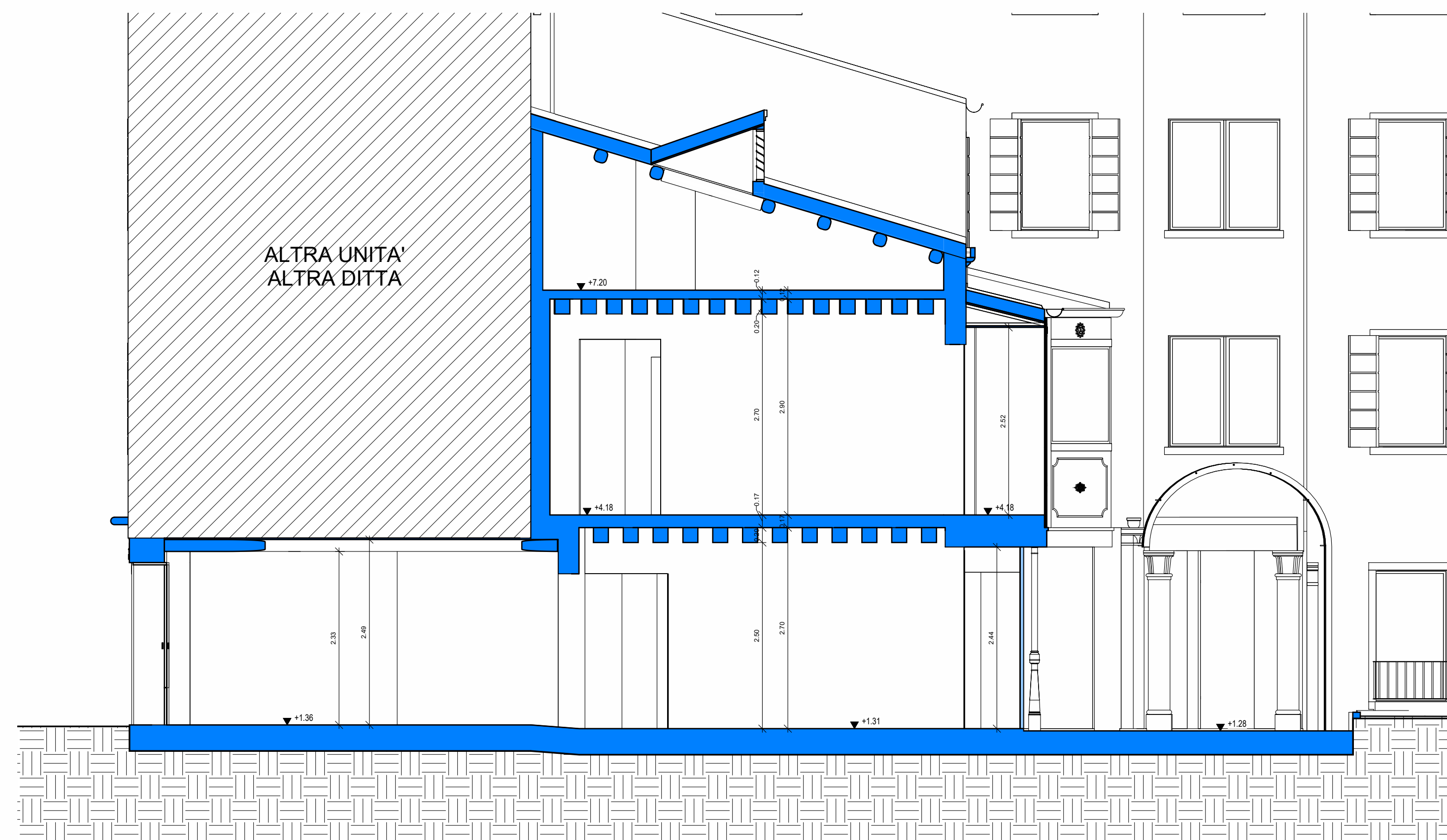
SEZIONE B-B - STATO DI PROGETTO
