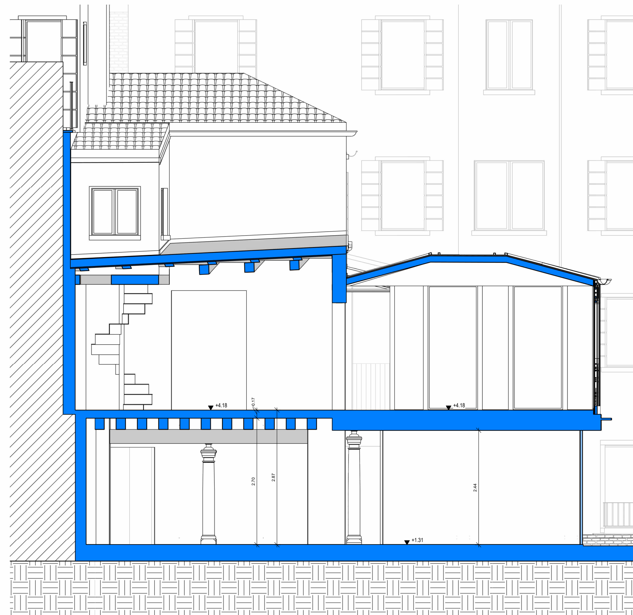
SEZIONE C-C - STATO DI PROGETTO
