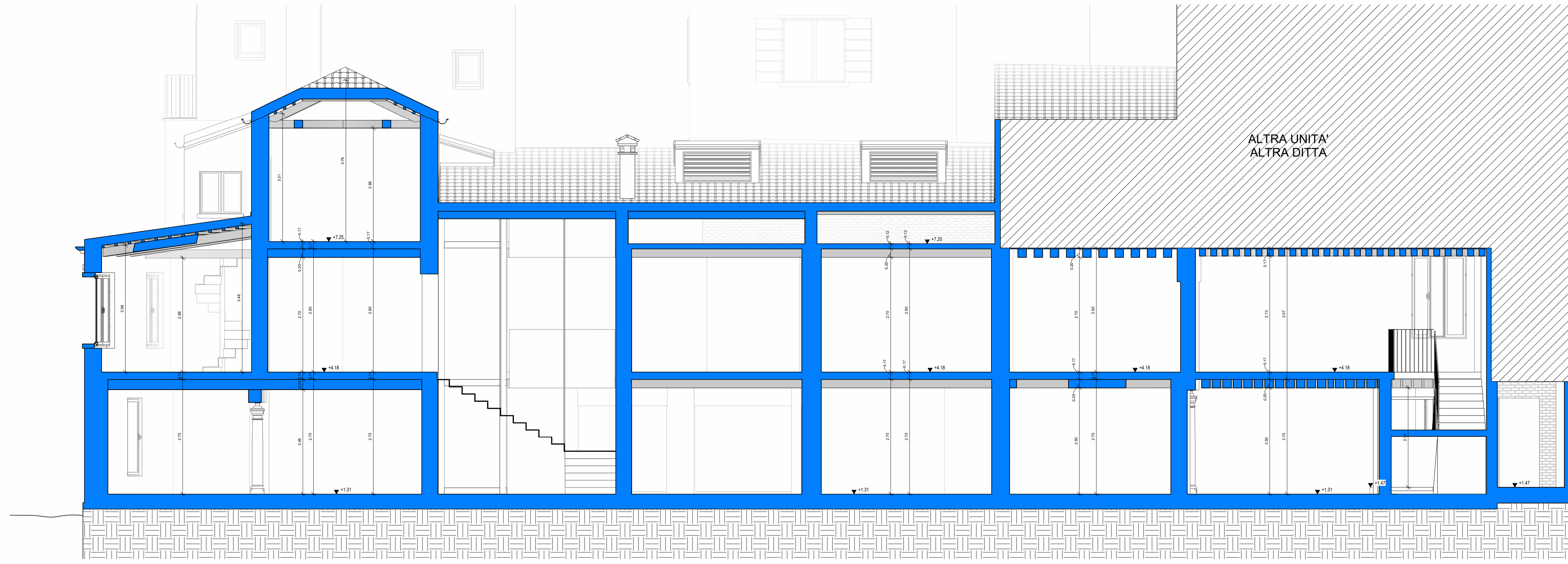
SEZIONE A-A - STATO DI PROGETTO
