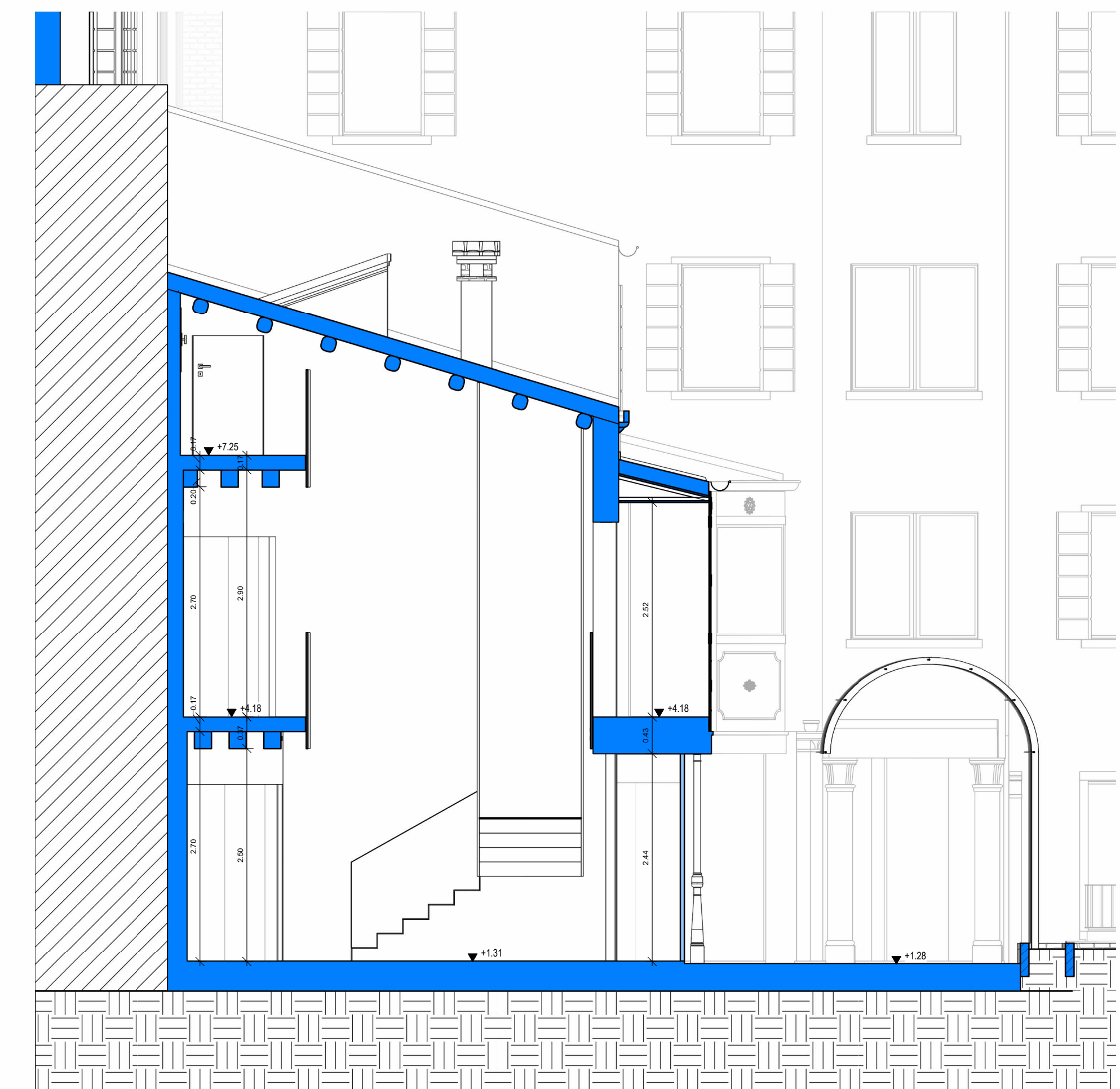
SEZIONE D-D - STATO DI PROGETTO
